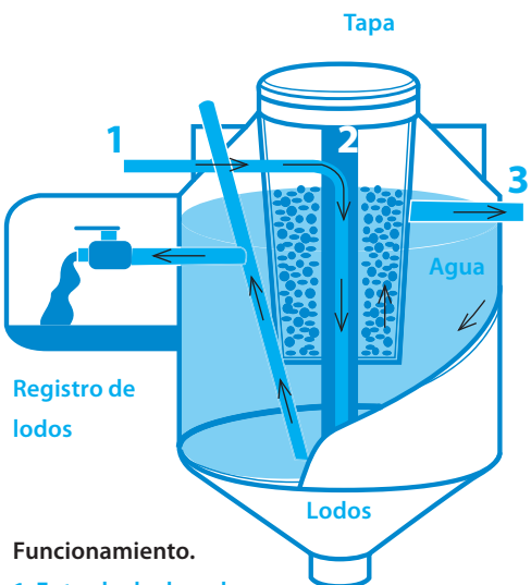
Instalación hidráulica.
